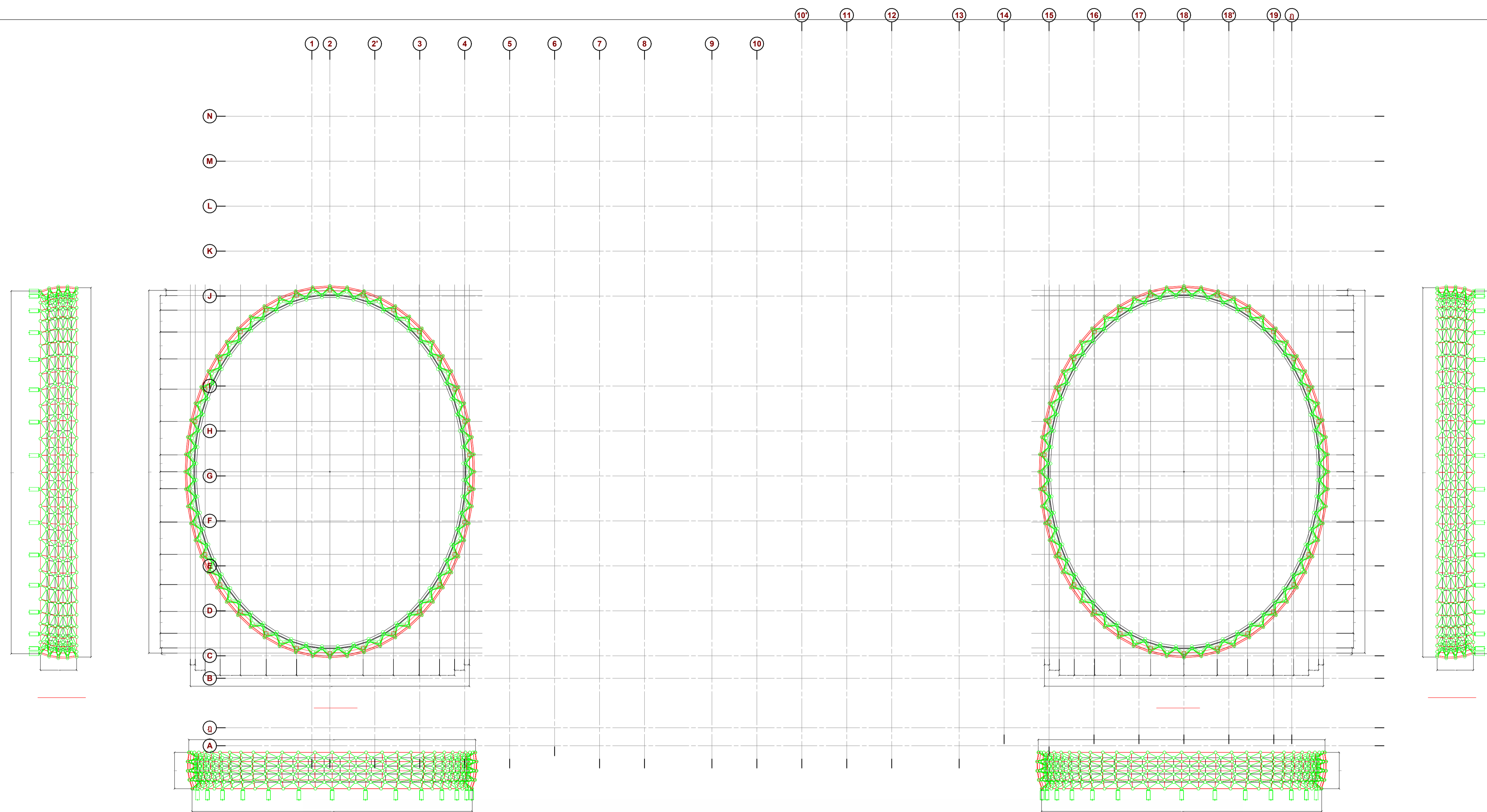
ผัง SPACE FRAME 2 SCALE 1 : 250
